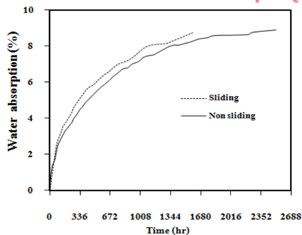
รูปที่ 1 ปริมาณการดูดซับน้ำของวัสดุเชิงประกอบพอลิไวนิลคลอไรด์ผสมผงซีลีเนียม
