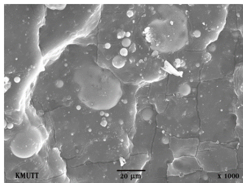
รูปที่ 2 ลักษณะพื้นผิวของอนุภาคเถ้าลอยในวัสดุผสมระหว่าง NR/SBR โดยกล้องจุลทรรศน์อิเล็กตรอนแบบส่อง กราด
